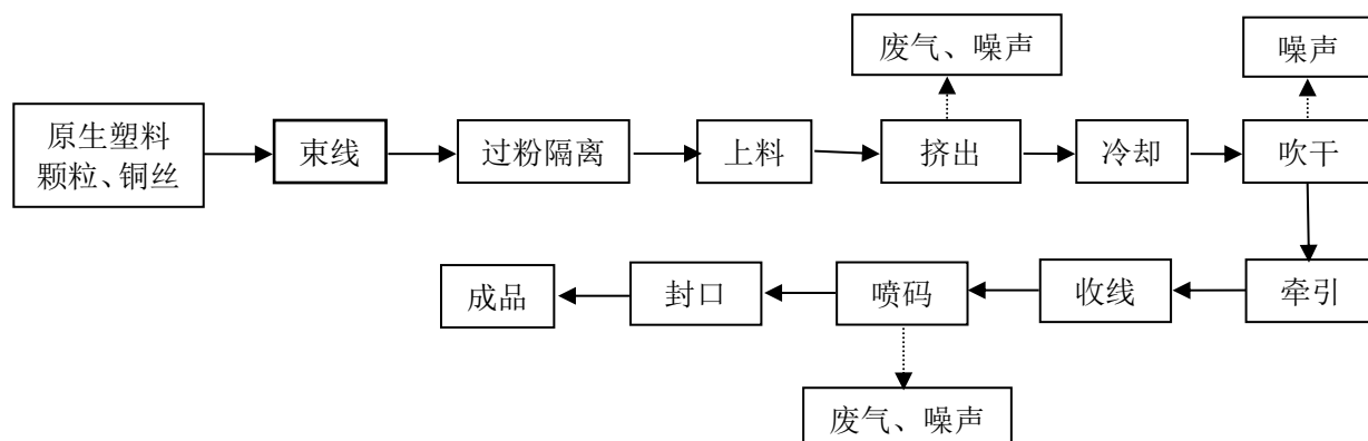
图 2-4 本项目生产工艺流程及产污环节图
