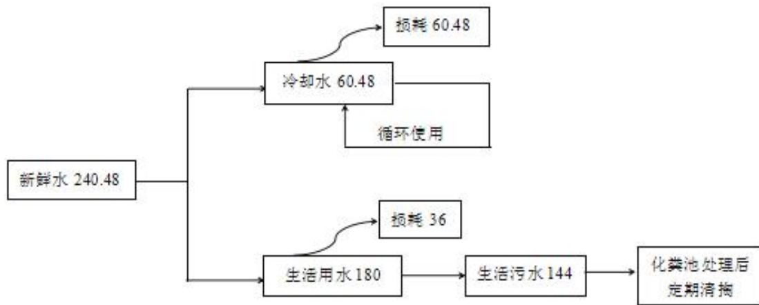
图 2-3 项目水平衡图 (m³/a)
